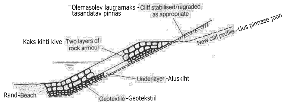
Joonis 3.1. Maakividest rannakindlustus erodeeruva nõlva kaitseks (CIRIA et al, 2007).
