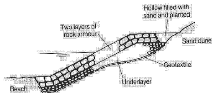
Joonis 3.2. Maakividest rannakindlustus eelluidete ja liivaranna kaitseks (CIRIA et al, 2007).
