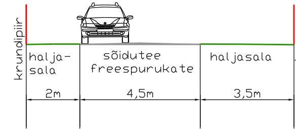
Planeeritud tänava lõige A-A'
