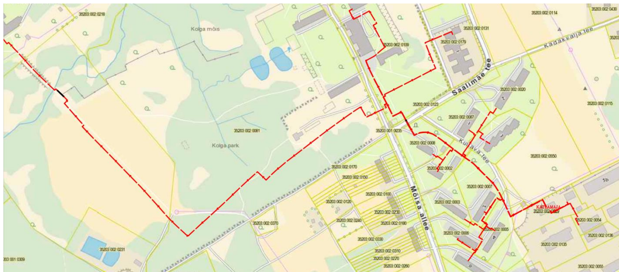
Joonis 16. Kolga kaugküttevõrgu skeem
