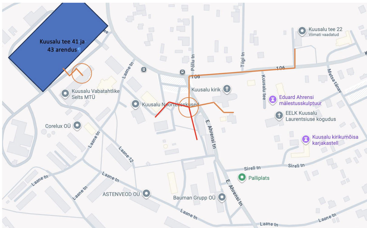
Joonis 12. Perspektiivse kaugkütetorustiku (tähistatud oranži joonega) paiknemise eskiis potentsiaalsete tarbijate liitmiseks (tähistatud oranži ringiga) olemasoleva kaugküttevõrguga (tähistatud punase joonega).
